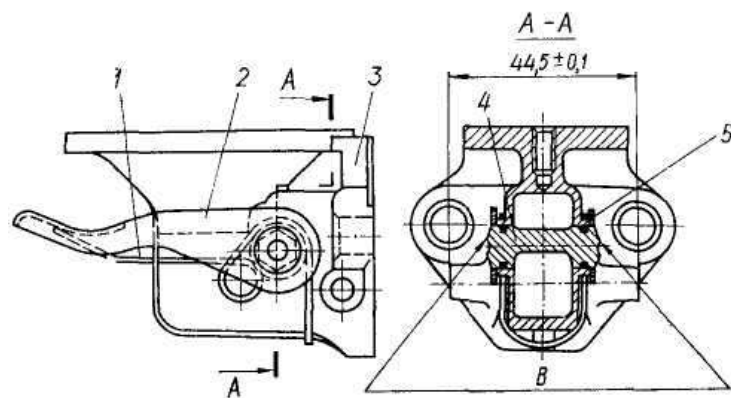
Рис. 34. Нижний корпус топливного насоса в сборе: 1 — пружина рычага; 2 — рычаг; 3 — нижний корпус; 4 — эксцентрик; 5 — кольцо уплотнительное; В — указанные места расклепать и заглаживать
