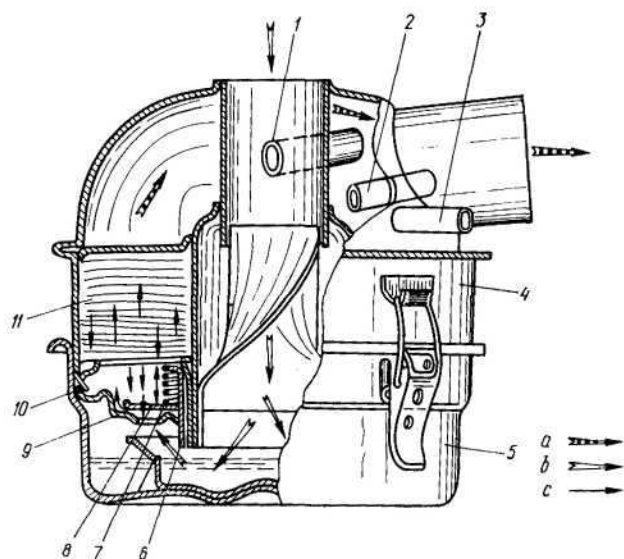
Рис. 40. Воздушный фильтр:
