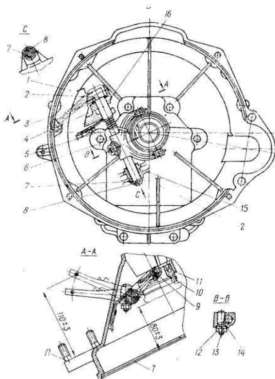
Рис. 106. Механизм выключения сцепления: 1 — картер сцепления; 2, 3 — нижняя и верхняя втулки оси; 4 — ось вилки с рычагом в сборе; 5 — возвратная пружина вилки выключения; 6 — вилка выключения; 7 — шайба регулировочная; 8 — пружинное кольцо; 9 — звено соединительное; 10 — подпятник; 11 — обойма подпятника; 12 — гайка; 13 — шайба пружинная; 14 — клин крепления вилки выключения сцепления фиксирующий; 15, 16 — нижний и верхний приливы
