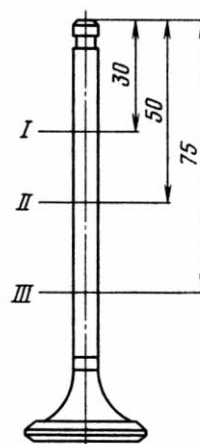
Рис. 80. Схема замера стержня клапана
