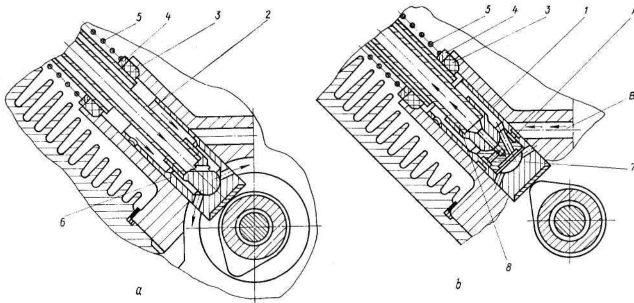
Рис. 19. Толкатели:
