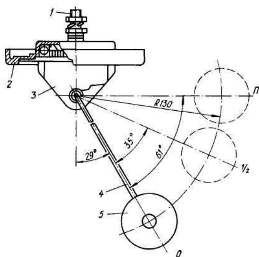
Рис. 234. Бензомер БМ136-А:
