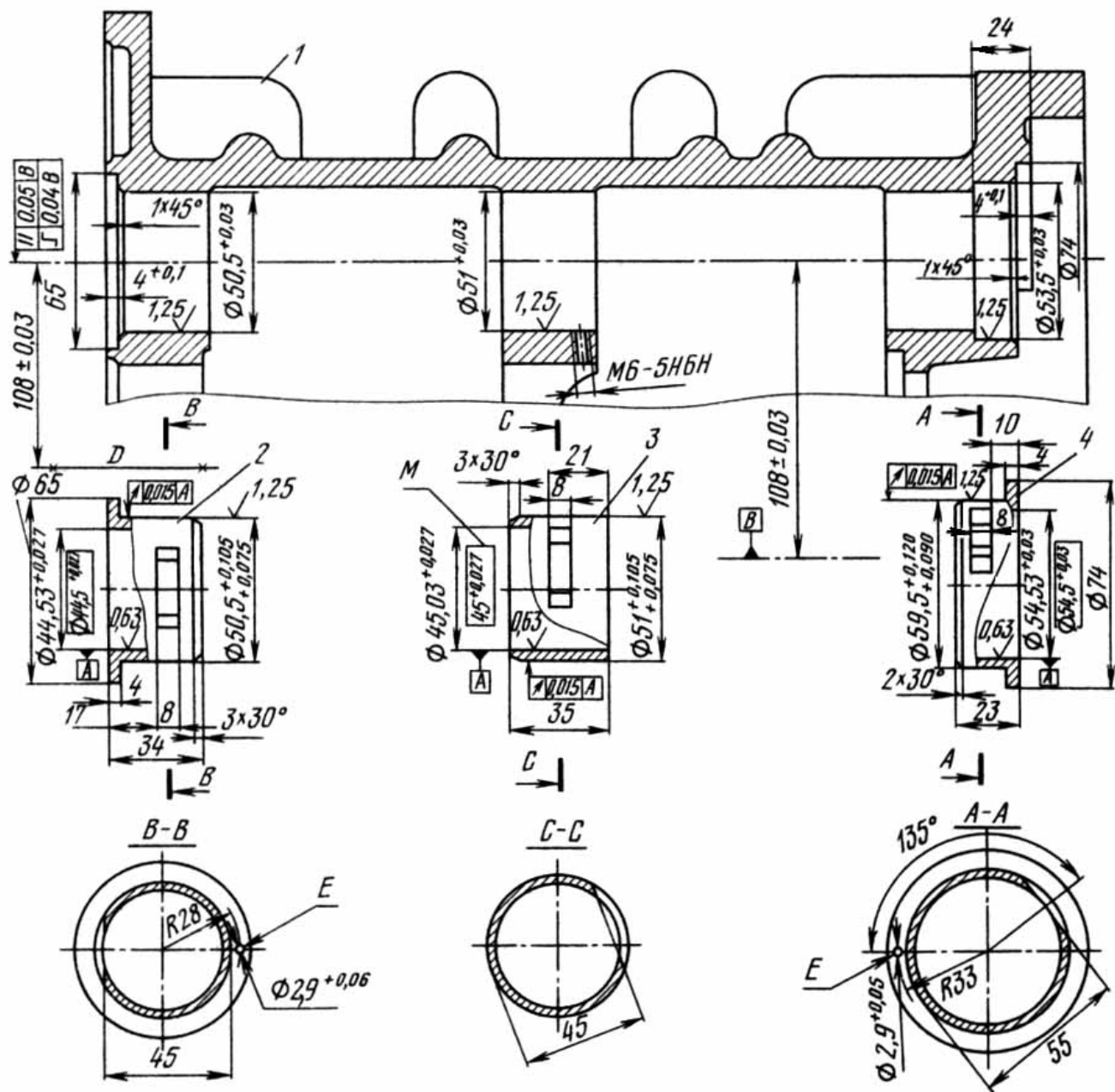
Рис. 65. Расточка картера двигателя под ремонтные подшипники распределительного вала: 1 — картер коленчатого вала; 2, 3, 4 — ремонтные подшипники опор распределительного вала; D — ось коленчатого вала
