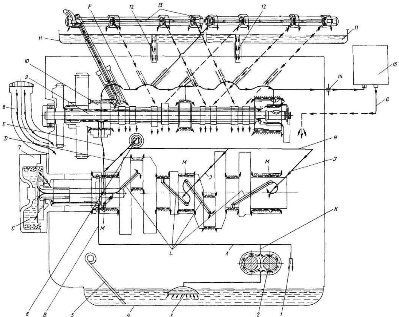
Рис. 23. Система смазки:
