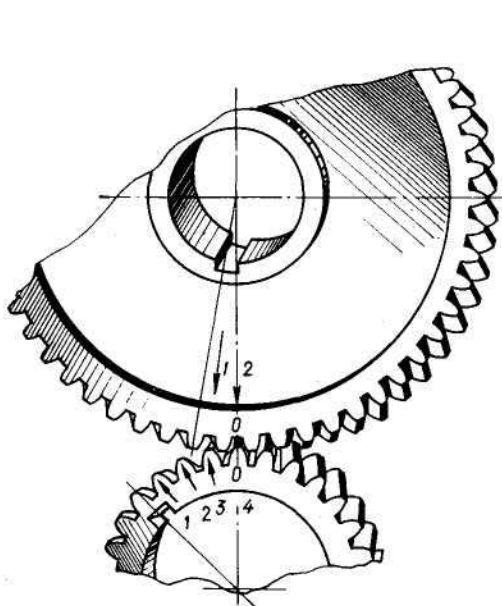
Рис. 14. Установочные метки O на распределительных шестернях
