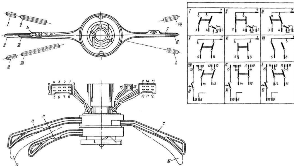
Рис. 220. Переключатель трёхрычажный:
