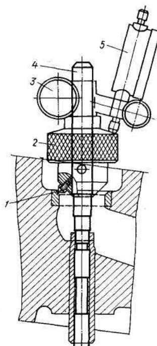
Рис. 85. Приспособление для проверки concentricity of the valve seat axis relative to the guide sleeve axis: 1 — шариковая головка; 2 — вращающаяся муфта; 3 — держатель; 4 — оправка; 5 — индикаторная головка
