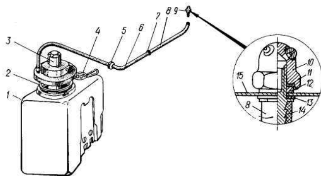
Рис. 239. Стеклоомыватель:
