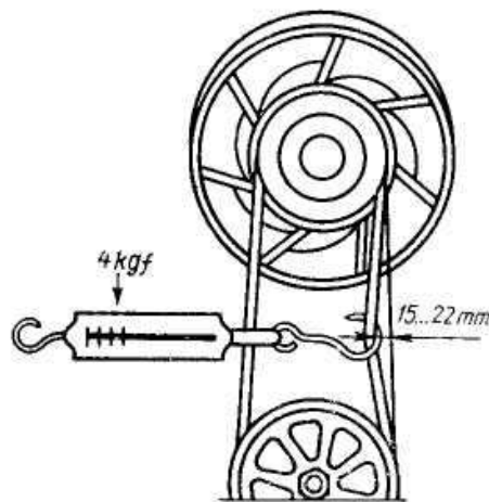
Рис. 99. Проверка натяжения ремня вентилятора
