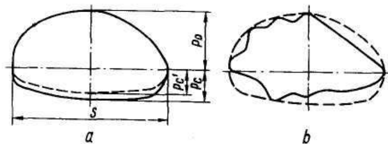
Рис. 182. Примерная форма диаграмм амортизаторов на специальном стенде:
