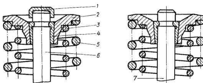
Рис. 21. Впускные и выпускные клапана:
