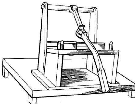
Рис. 77. Приспособление для снятия и установки пружин клапанов
