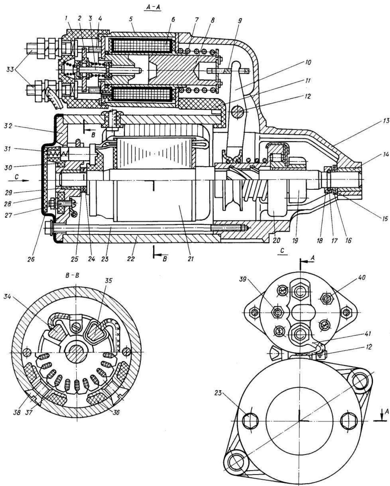
Рис. 215. Стартер СТ368:
