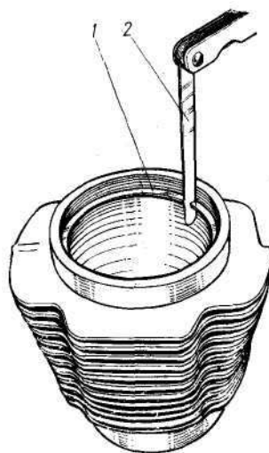
Рис. 72. Замер теплового зазора в стыке замка поршневого кольца, установленного в цилиндр: 1 — поршневое кольцо; 2 — щуп
