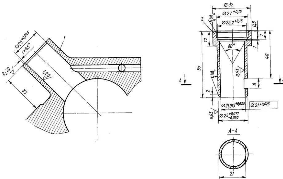
Рис. 66. Расточка картера двигателя под ремонтные втулки бонок толкателя: 1 — картер коленчатого вала; 2 — ремонтная втулка бонки толкателя
