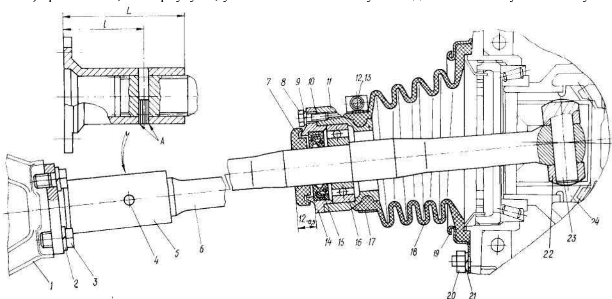
Рис. 151. Полуось:
