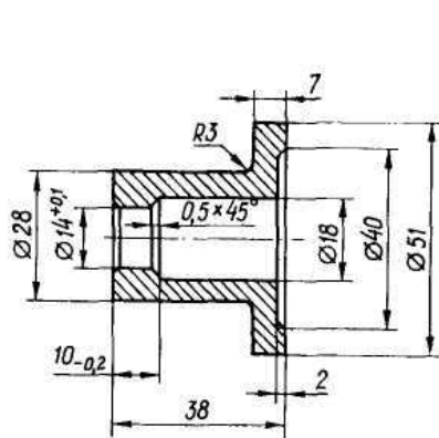
Рис. 163. Оправка для выпрессовки и запрессовки наружного подшипника ведущего вала колёсного редуктора
