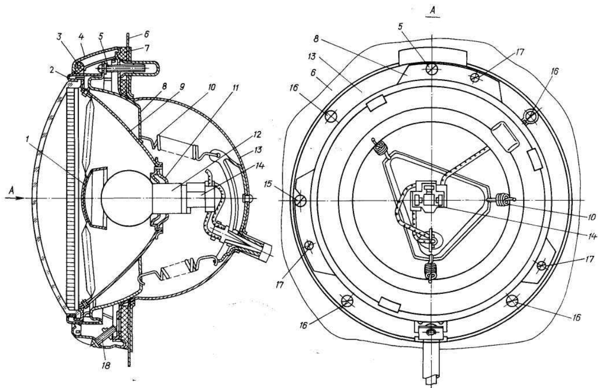
Рис. 222. Фара:
