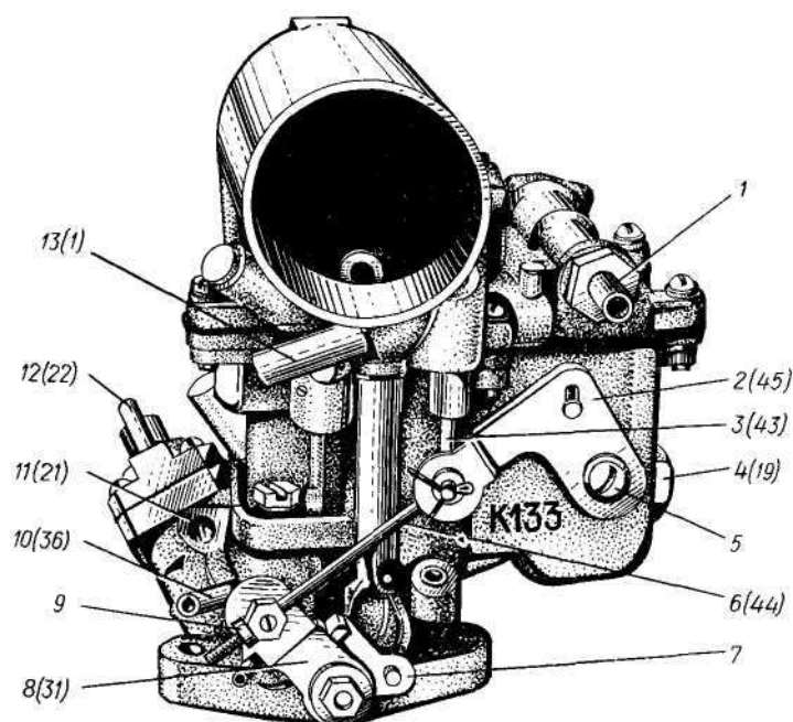
Рис. 37. Карбюратор K133; вид сзади (в скобках указаны номера позиций данных деталей на схеме карбюратора (рис. 35)):
