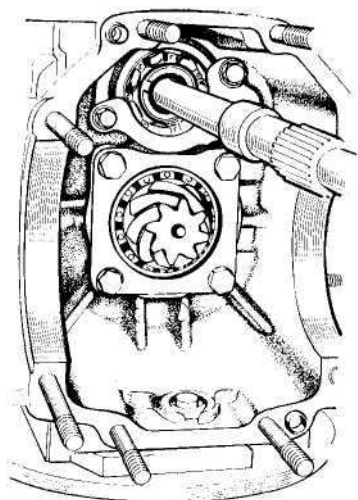
Рис. 139. Вид со стороны ведущего вала
