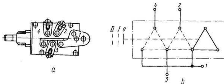
Рис. 219. Центральный переключатель света ПЗ05:
