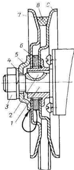
Рис. 98. Устройство для натяжения, ремня вентилятора: 1 — вал генератора; 2 — шпонка; 3 — гайка; 4 — шайба; 5 — нажимной колпачок; 6 — шайбы регулировочные; 7 — передняя половина шкива; 8 — ремень; 9 — задняя полови- на шкива
