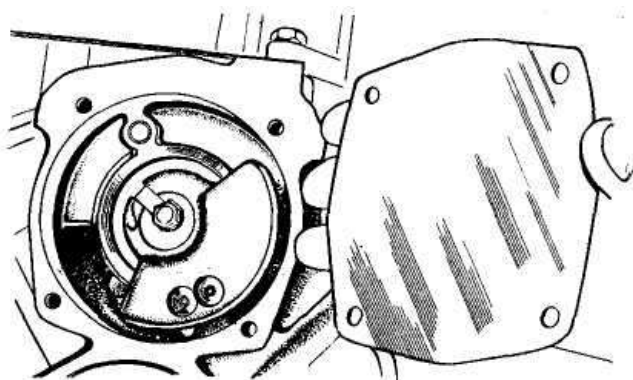
Рис. 59. Вид на балансир со стороны маховика при снятой крышке балансиного вала
