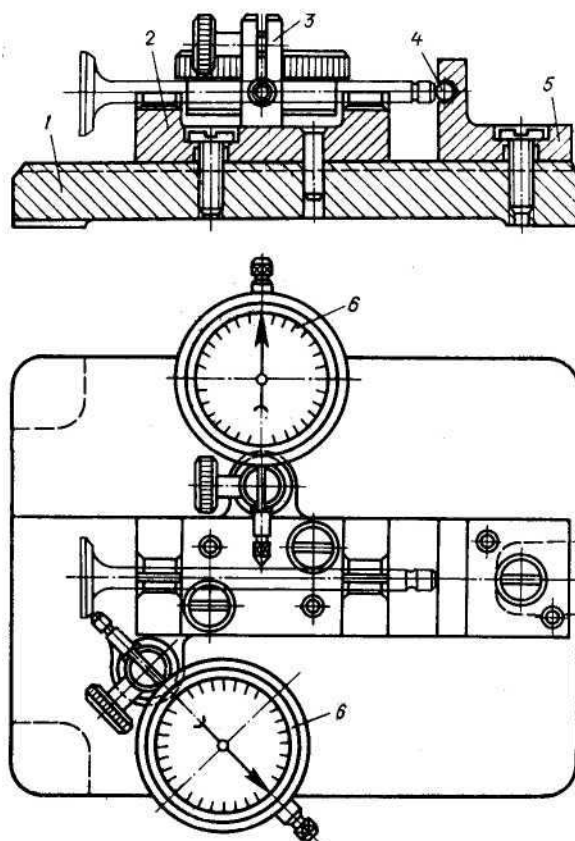
Рис. 83. Проверка клапана на concentricity рабочей фаски головки и стержня: 1 — плита; 2 — призма; 3 — держатели; 4 — шарик; 5 — стойка; 6 — индикатор
