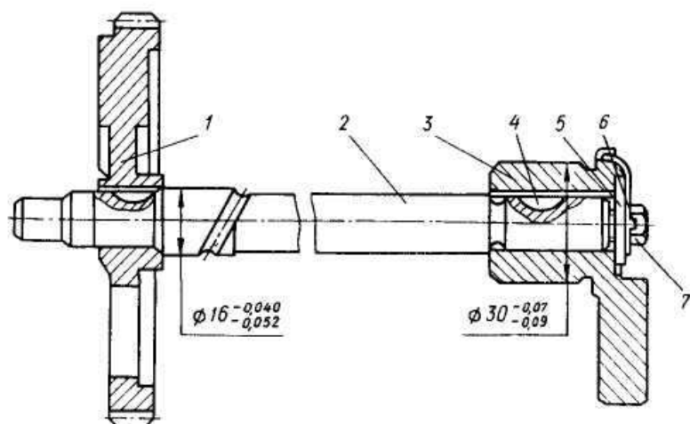
Рис. 16. Механизм балансирный в сборе: 1 — шестерня балансирного вала; 2 — вал балансирный; 3 — балансир; 4 — шпонка сегментная; 5 — шайба балансирного вала; 6 — шайба стопорная; 7 — болт
