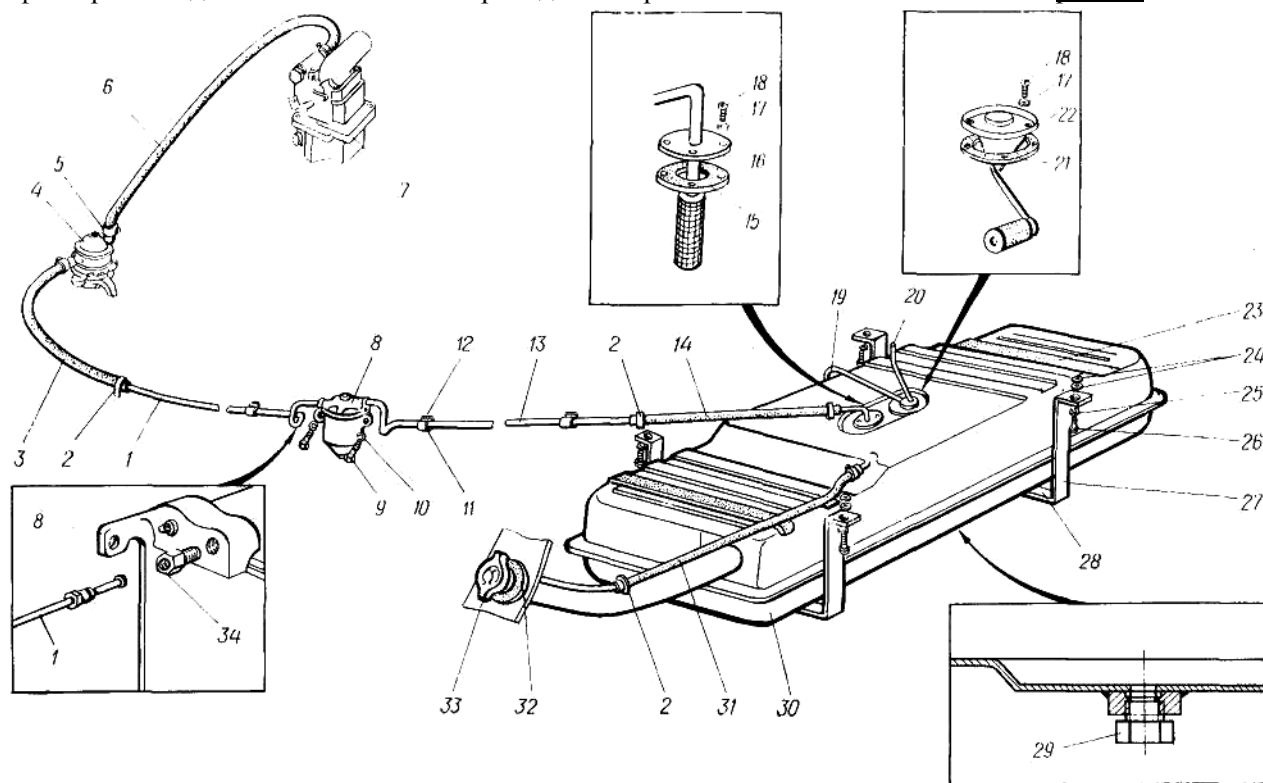
Рис. 30. Система питания:
