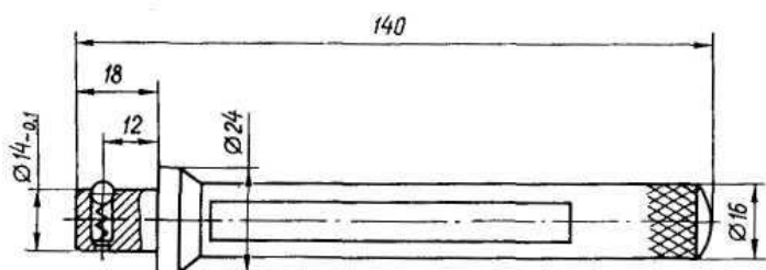
Рис. 157. Ручка оправок
