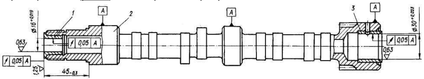
Рис. 13. Вал распределительный в сборе:
