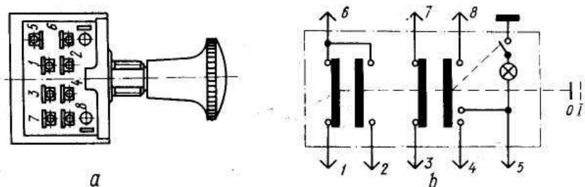
Рис. 229. Выключатель аварийной сигнализации:
