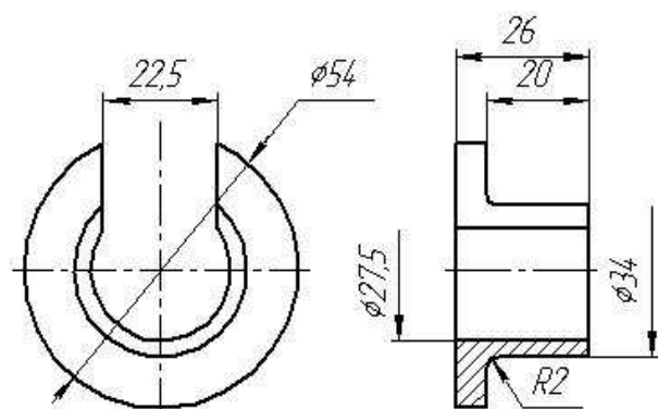
Рис. 154. Оправка для спрессовки подшипникового узла с полуоси
