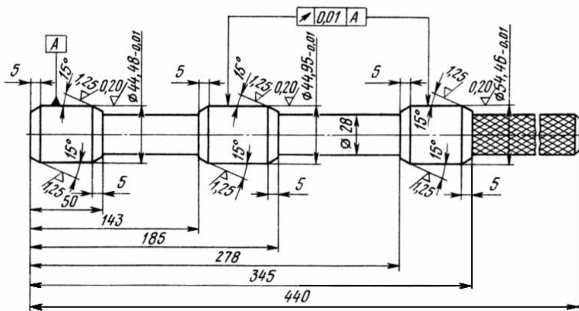
Рис. 67. Оправка для проверки соосности подшипников распределительного вала
